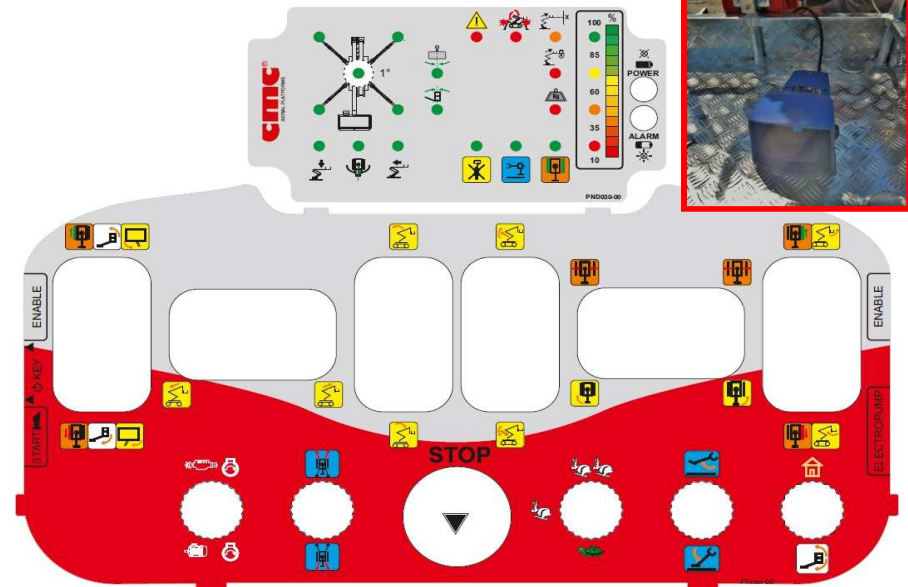
Figure 12 : poste de commande du panier + pédale à action maintenue.
