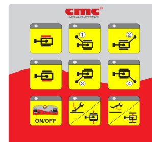
Figure 48 : poste de commande stabilisateurs.
