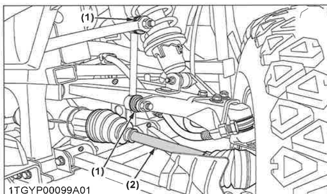
1TGYP00099A01 (1) Stofhoes (2) Voorste aandrijfjas
