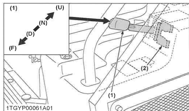
(1) Hendel hydraulische hefcilinder (D) „OMLAAG” (F) „ZWEEFSTAND met vergrendeling” (2) Begrenzingsplaat (U) „OMHOOG” (N) „NEUTRAAL”
