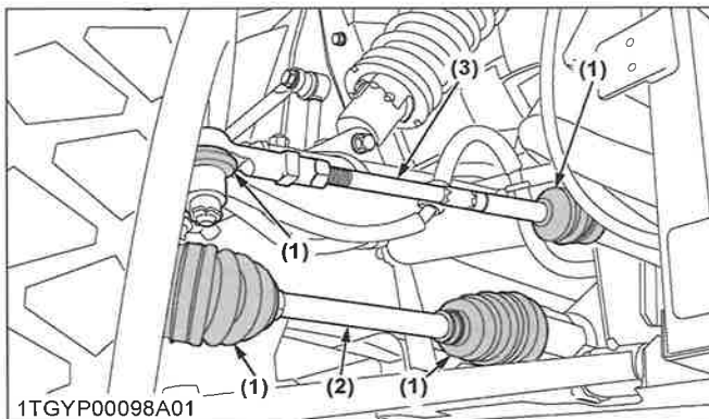
1TGYP00098A01 (1) Stofhoes (2) Voorste aandrijfjas (3) Trekstang
