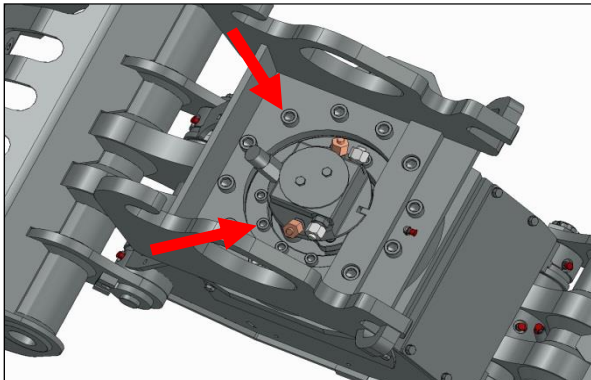
Fig. 12: Draaikrans bouten
